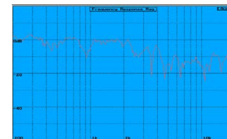
Réponse en fréquence de 200Hz à 20 kHz à 60° pour 8 V
