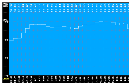
Réponse en fréquence en 1/3 octave pour 8 V
