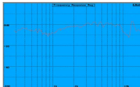
Réponse en fréquence de 200Hz à 20 kHz dans l'axe pour 8 V
