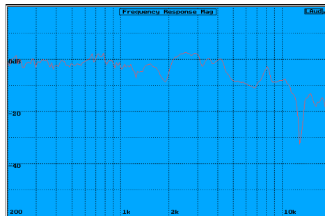
Réponse en fréquence de 200Hz à 20 kHz dans l'axe
