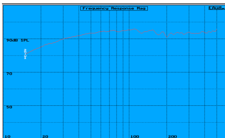
Réponse en fréquence en champ proche
